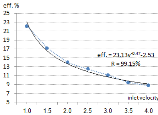
Hình 4.5. Tương quan giữa hiệu suất truyền nhiệt eff. và vận tốc inlet m/s
